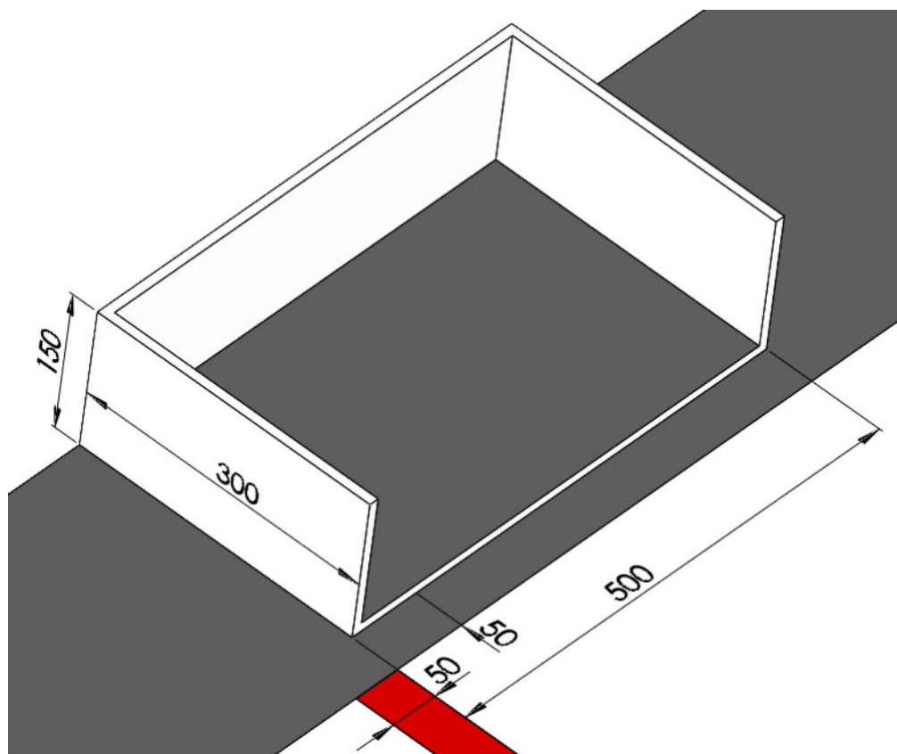
图 6 住户标识尺寸（单位：mm）
