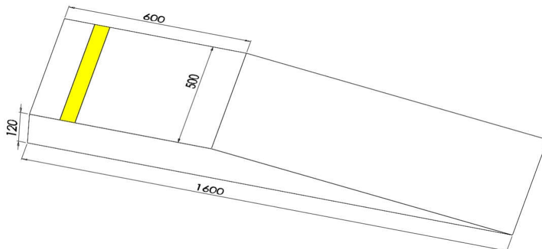
图4 高台和斜坡尺寸（单位：mm）
