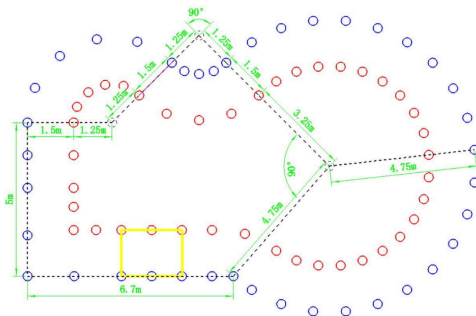
图2 赛道俯视图及各指标尺寸
