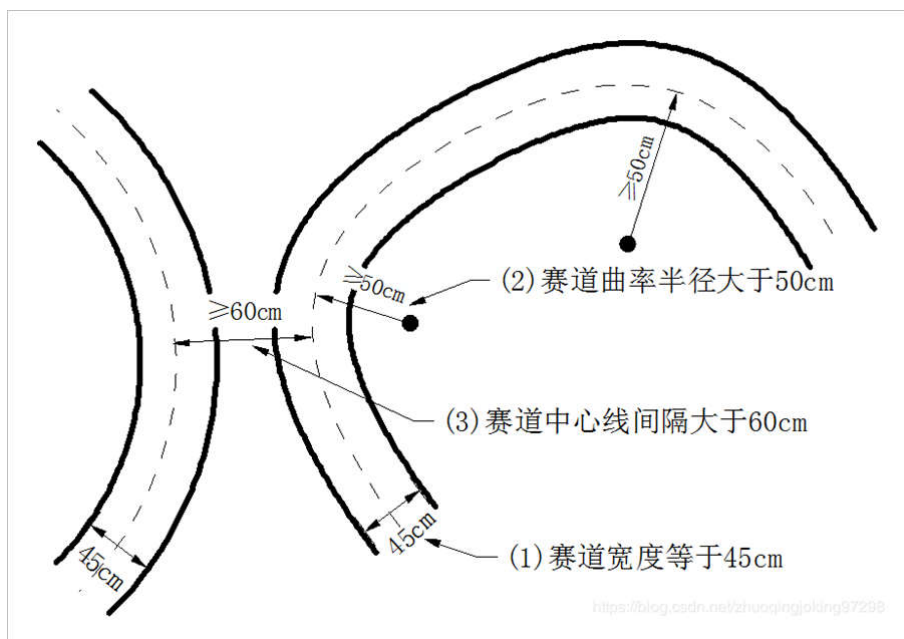
图 1 赛道基本尺寸
