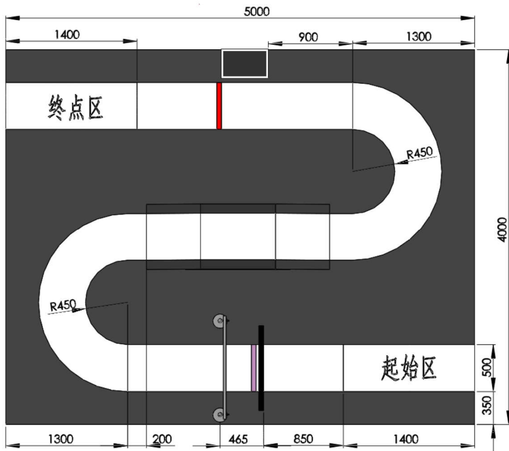
图 2 比赛场地整体尺寸 (单位: mm)
