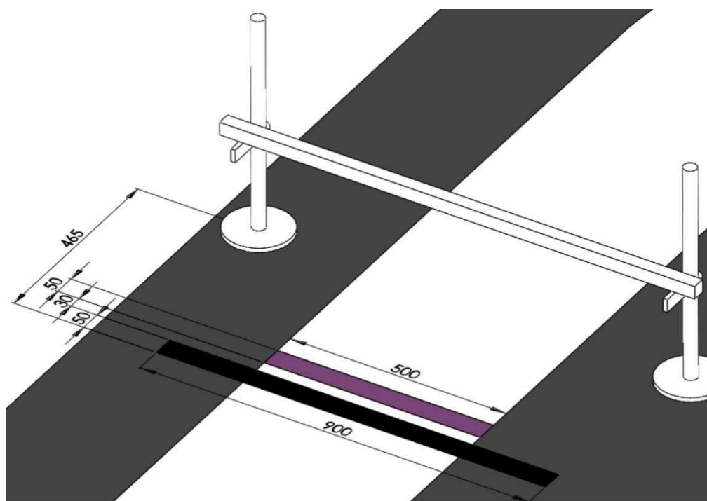
图5 限高杆辅助提示图（单位：mm）
