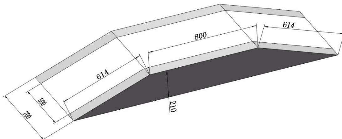
图4 上下斜坡尺寸（单位：mm）
