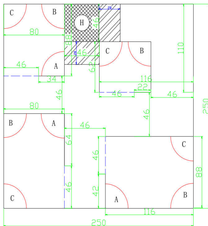
图 1 比赛场地平面图(单位:cm)
