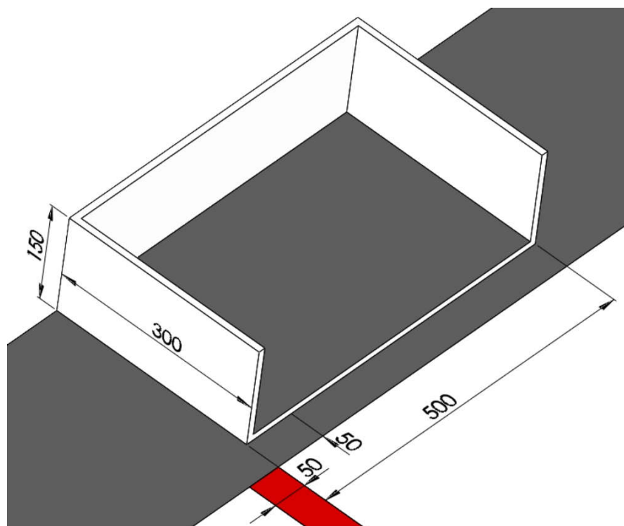
图 6 住户标识尺寸（单位：mm）
