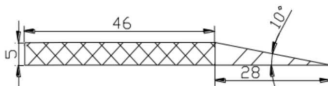
图 2 启动区平台斜坡示意图(单位:cm)
