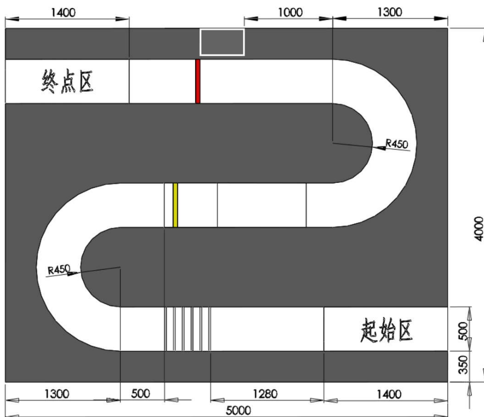
图 2 比赛场地整体尺寸 (单位: mm)
