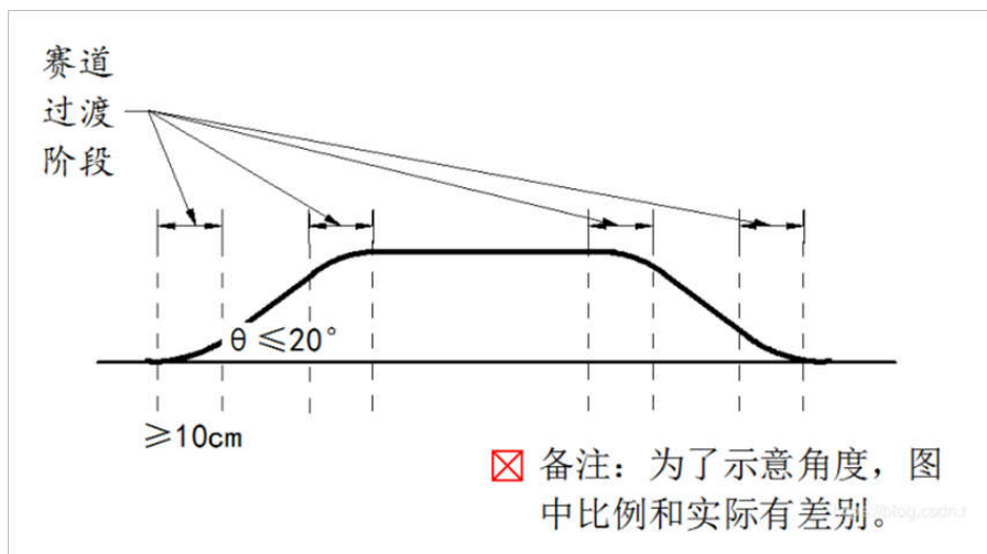
图3 坡道示意图
