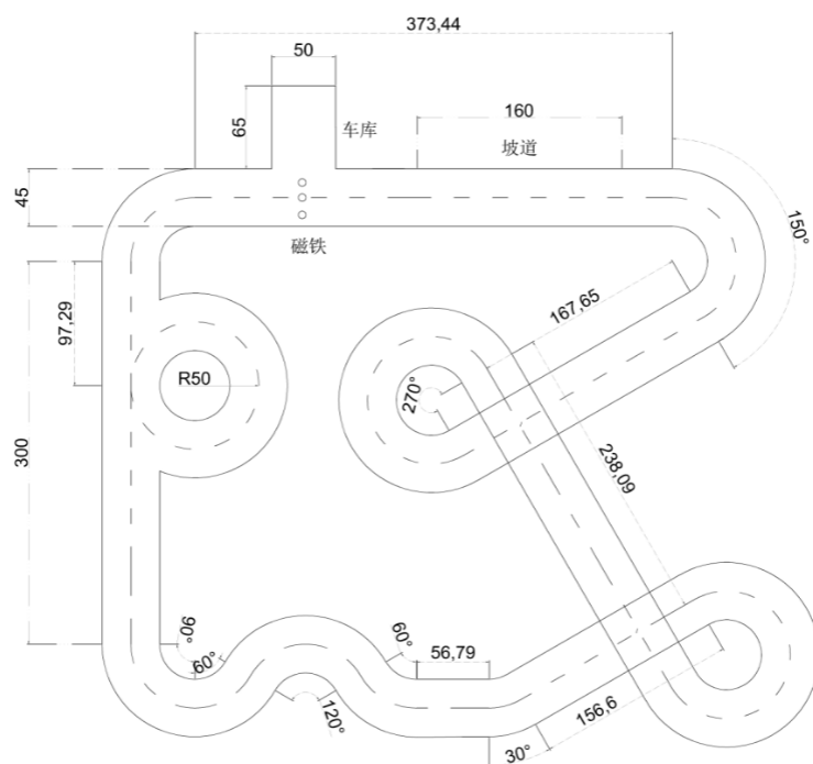
图 1 比赛赛道
