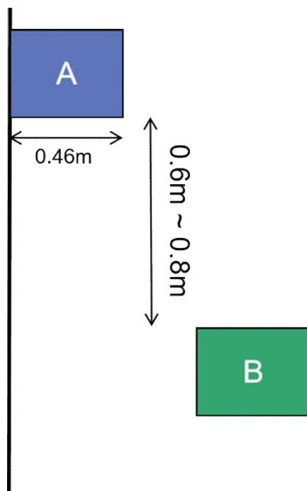
图 6 避障设计图
